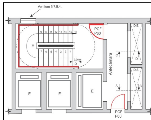
Figura 9 - Escada enclausurada à prova de fumaça
