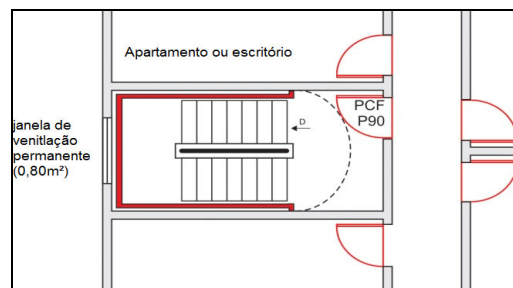
Figura 7 - Escada enclausurada protegida
