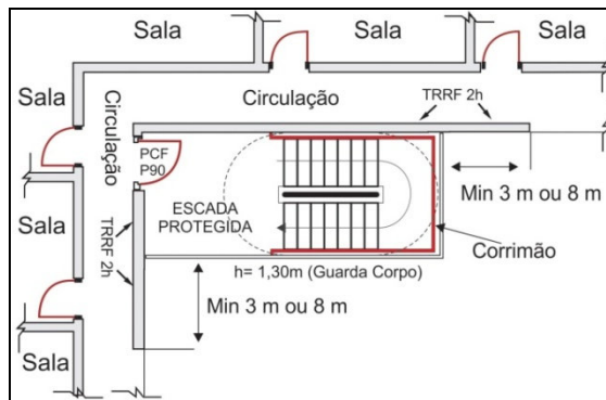
Figura 13 - Escada aberta externa
