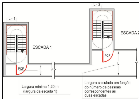
Figura 19 - Dimensionamento de corredores de descarga
